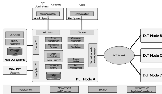
(그림 1) DLT 시스템 기능 요소
