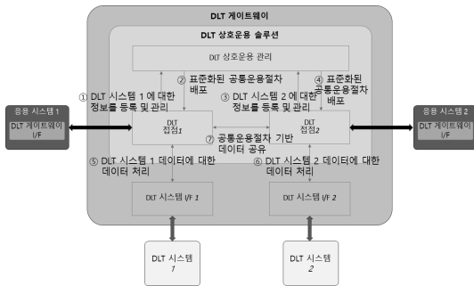
(그림 12) DLT 게이트웨이 운영 절차
