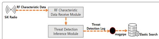
(그림 4) 위협 탐지 에이전트 프로세스 (Figure 4) Threat detection agent process
