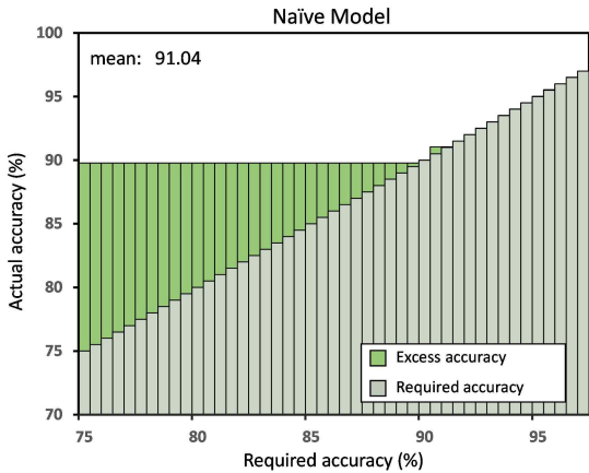
그림 5. 전체 탐색 기법의 요구사항에 따른 정확도 성능
