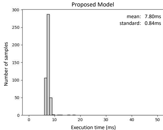
그림 4. 제안 기법의 수행 시간
