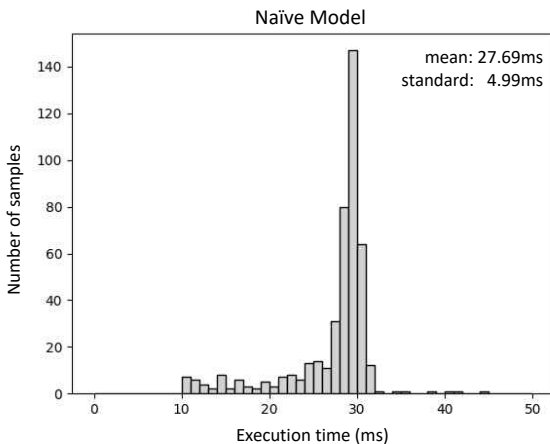
그림 3. 전체 탐색 기법의 수행 시간
