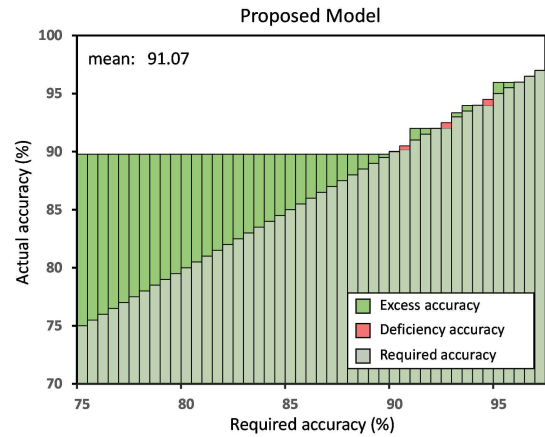
그림 6. 제안 기법의 요구사항에 따른 정확도 성능
