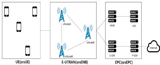
그림 1 srsLTE 도식도
