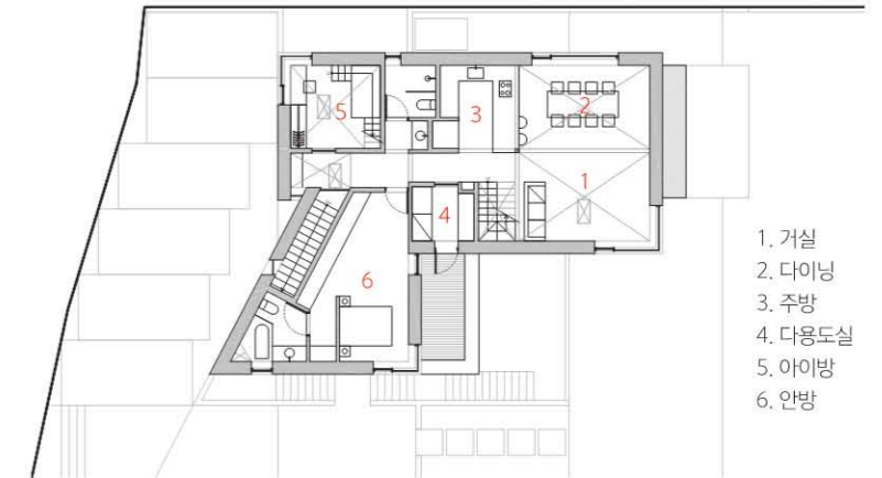
2층 평면도
