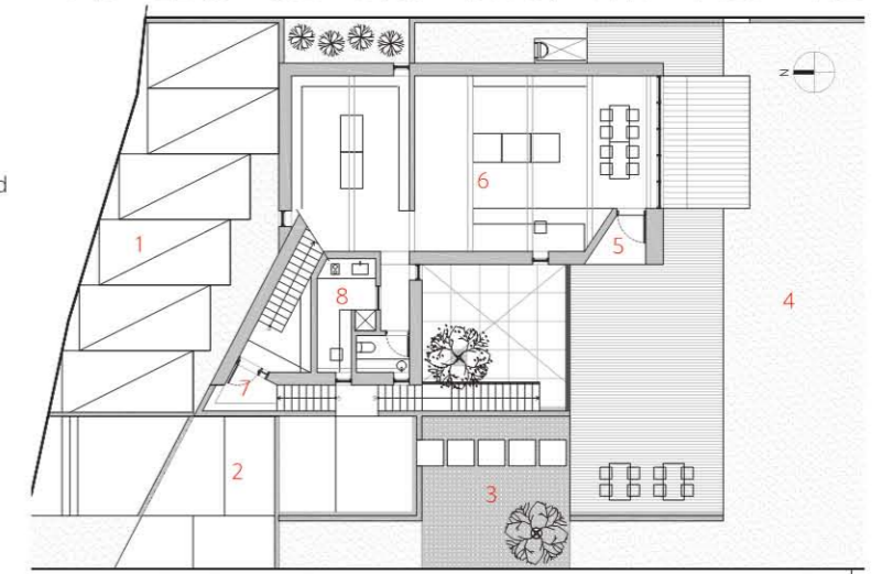
1층 평면도
