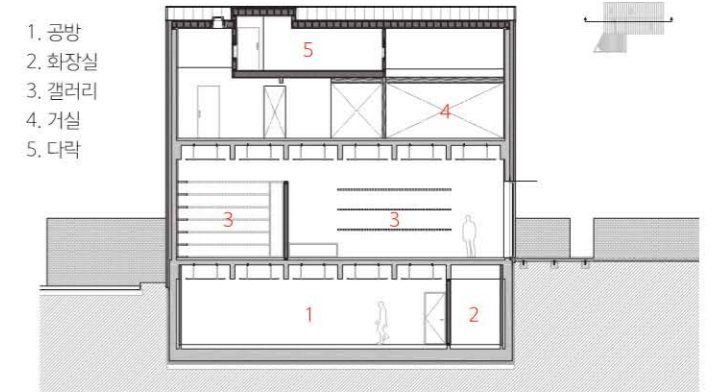
단면도
