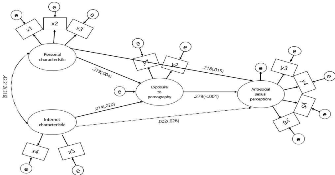
그림 2. 수정모형의 경로계수
