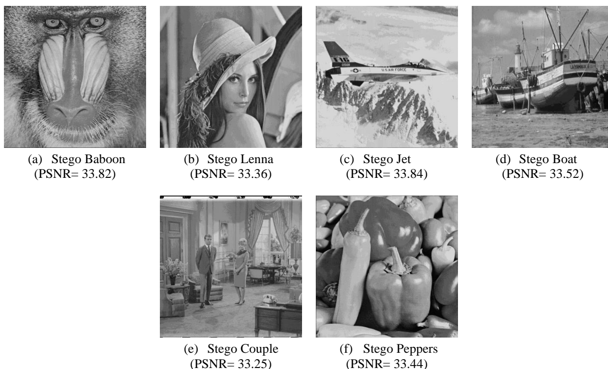
Fig. 6. Stego Images
