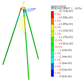
(d) Bending moment diagram (Y-direction)
