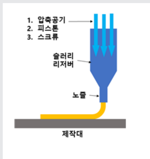
그림 5. DW 3D 프린팅 모식도
