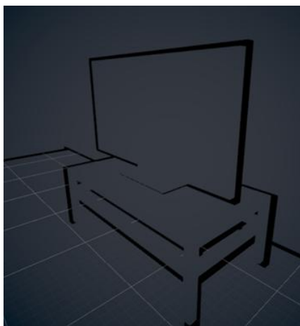
Fig. 5. Outline Shader
