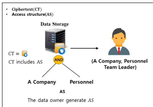
Fig. 2. CP-ABE
