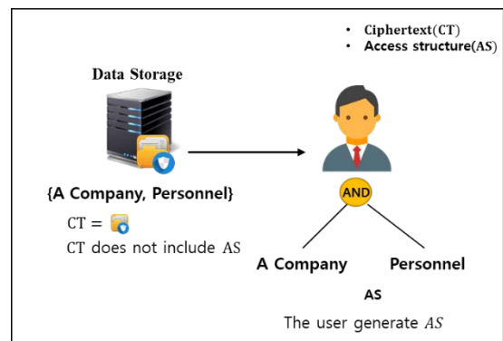
Fig. 3. KP-ABE
