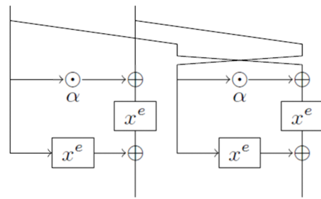
(그림 6) 닫힌 버터플라이(Closed Butterfly) 구조
