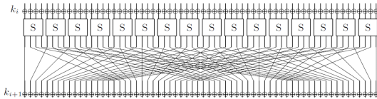
(그림 2) 블록암호 PRESENT의 라운드 함수
