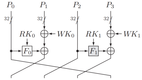
(그림 3) 블록암호 CLEFIA의 라운드 함수
