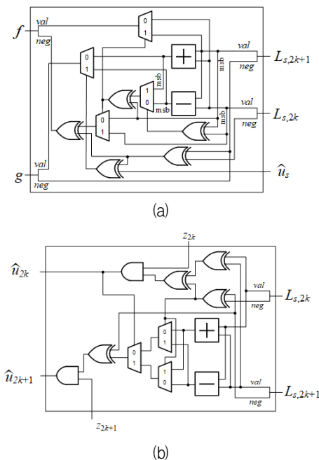
Fig. 7. (a) PE architecture and (b) P architecture of Redundant-LLR SC decoder for polar code when N = 8 [15]. 그림 7. N = 8 일때 redundant-LLR 기반의 연속 제거 복호기의 (a) PE 구조와 (b) P 구조 [15]
