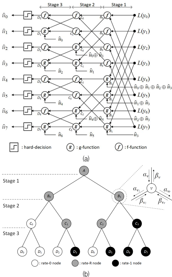
Fig. 1. (a) SC decoding procedure [1] and (b) decoding tree for (8, 4) polar code. 그림 1. (8, 4) polar code의 (a) 연속 제거 복호 과정 [1]과 (b) 복호 트리
