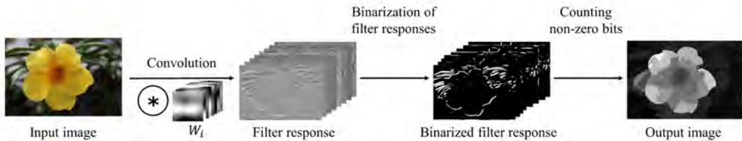
그림 3. 이진 통계 영상 특징 표현자를 이용한 흐려짐 검출 Fig. 3. Overview of blur detection using the binarized statistical image feature
