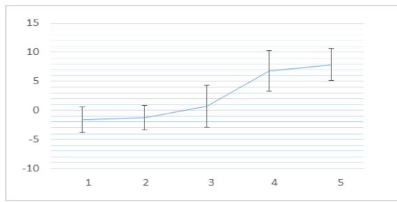
그림 2. 지각에 따른 피치편차의 평균값(Qt) Figure 2. Perceptual rating and pitch differences between boundary and penultimate syllables
