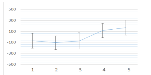
그림 1. 지각과 경계성조의 기울기(Hz/ms) Figure 1. Perceptual rating and slope of boundary tones
