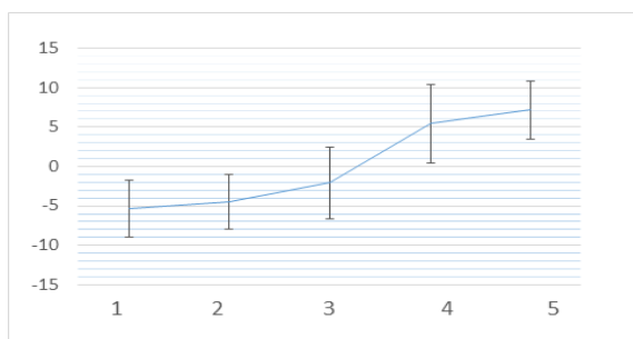
그림 3. 지각에 따른 피치레벨의 평균값(Qt) Figure 3. Perceptual rating and pitch level of boundary tones
