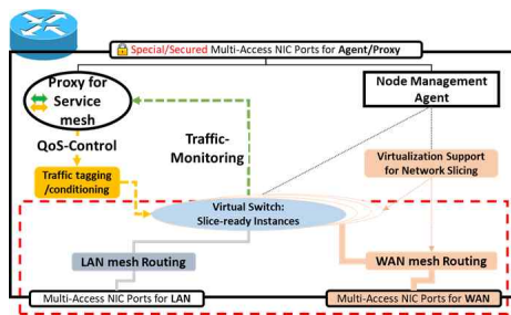
그림 5. 전술메쉬 WAN 노드 개념설계의 가상화 기반 네트워크 (요구사항 R1)
