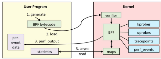
그림 8. Linux eBPF의 동작방식[12]
