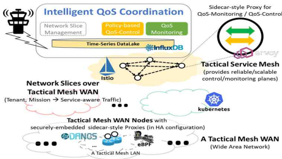
그림 2. 오픈소스 소프트웨어를 활용한 소프트웨어 중심 미래형 전술메쉬망의 시험적인 설계방안
