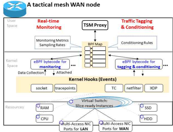
그림 9. 전술메쉬 WAN 노드를 위한 eBPF 기반 실시간 모니터링 설계
