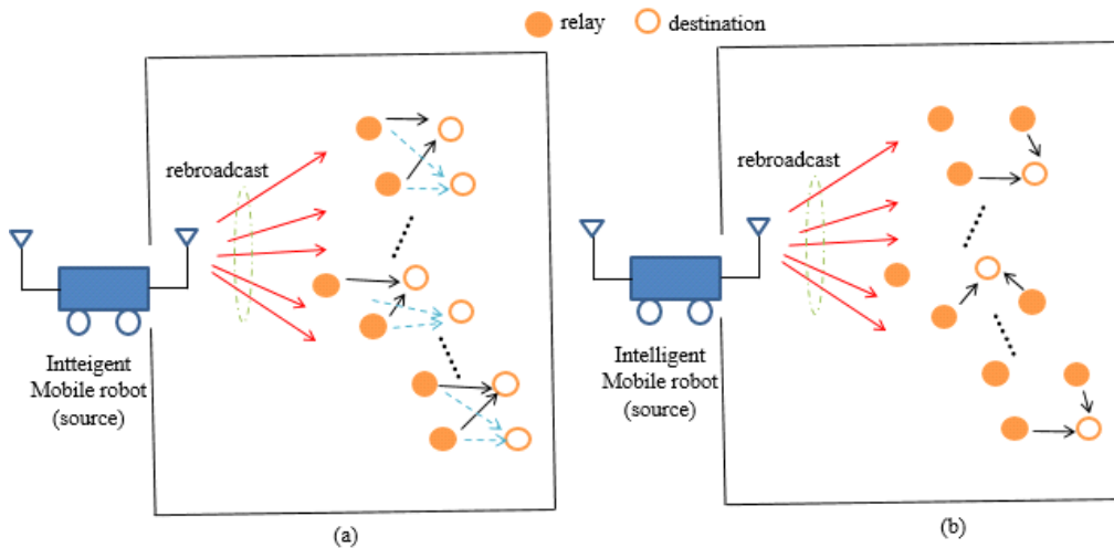
그림 3. 지능형 이동 로봇들 간의 협업을 위한 제안된 협력통신 방식 Fig. 3. The proposed cooperative communications for the collaboration of intelligent mobile robots
