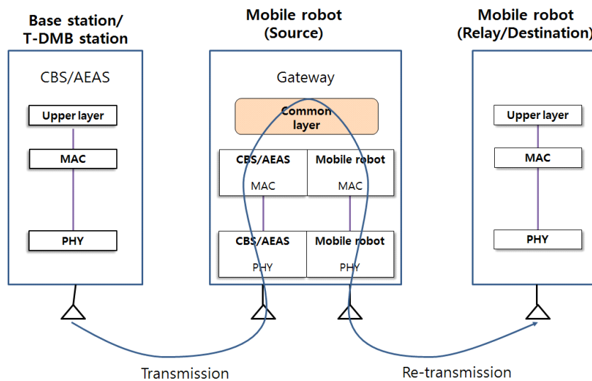
그림 2. 재난경보 방송의 재전송을 위한 지능형 이동 로봇 제공원의 게이트웨이 구조 Fig. 2. The gateway structure of the intelligent mobile-robot source for re-transmission of emergency alert broadcast
