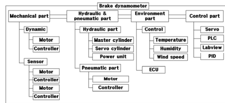
Fig. 4. Brake dynamometer diagram
