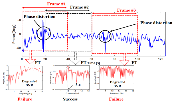
그림 6. 실시간 생체신호 탐지를 위한 구조 Fig. 6. Framework for real-time vital sign detection.
