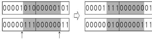
〈Figure 9〉 Multi Point Crossover
