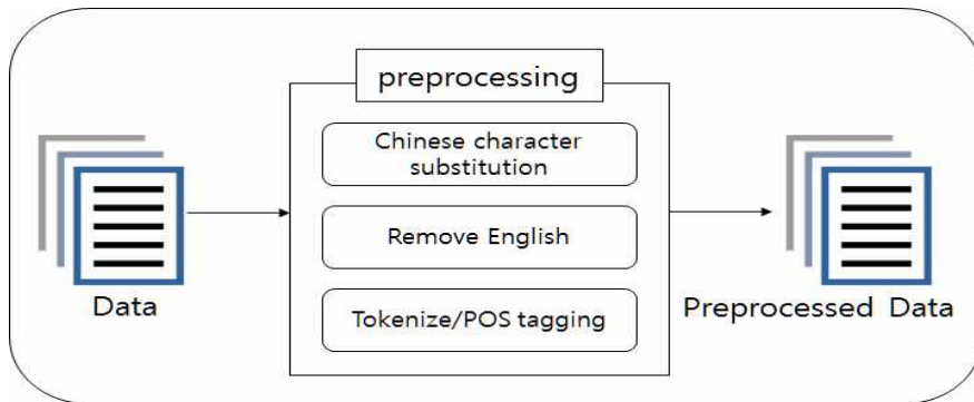
그림 3. 문서 분류기의 데이터 전처리 과정 Fig. 3. Document classification data preprocessing
