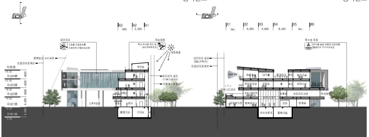
중단면도
