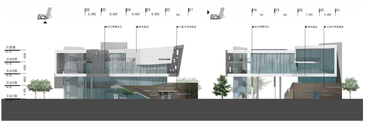
북측면도
