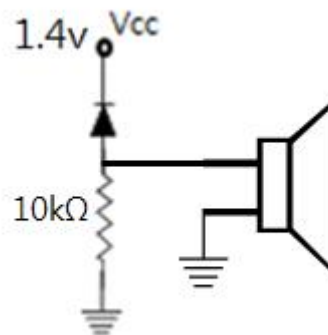
그림 6. 아날로그 방식 수신 모듈 회로도
