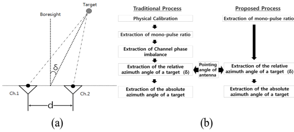
그림 2. (a) 모노펄스 시스템의 표적 방위각 모식도, (b) 표적 방위각 추출절차 Fig. 2. (a) Diagram of target azimuth angle for mono-pulse system, (b) Extraction procedure of target azimuth angle.
