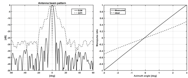
(a) 안테나 빔패턴(실선: 합 채널, 점선: 차 채널) (a) Antenna beam pattern(real line: Sum channel, dotted line: Diff. channel.) (b) 모노펄스 기울기(실선: 측정결과, 점선: 이상적 경우) (b) Mono-pulse ratio(real line: measured, dotted line: ideal case)
