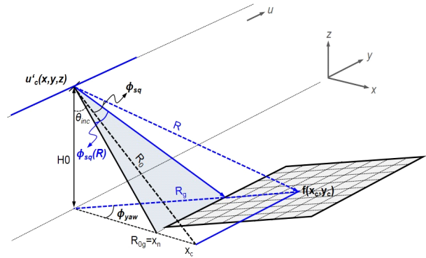
그림 2. Squint-SAR 시스템의 방위각 성분 분석 Fig. 2. Geometry of squint-SAR system for analyzing azimuth components.
