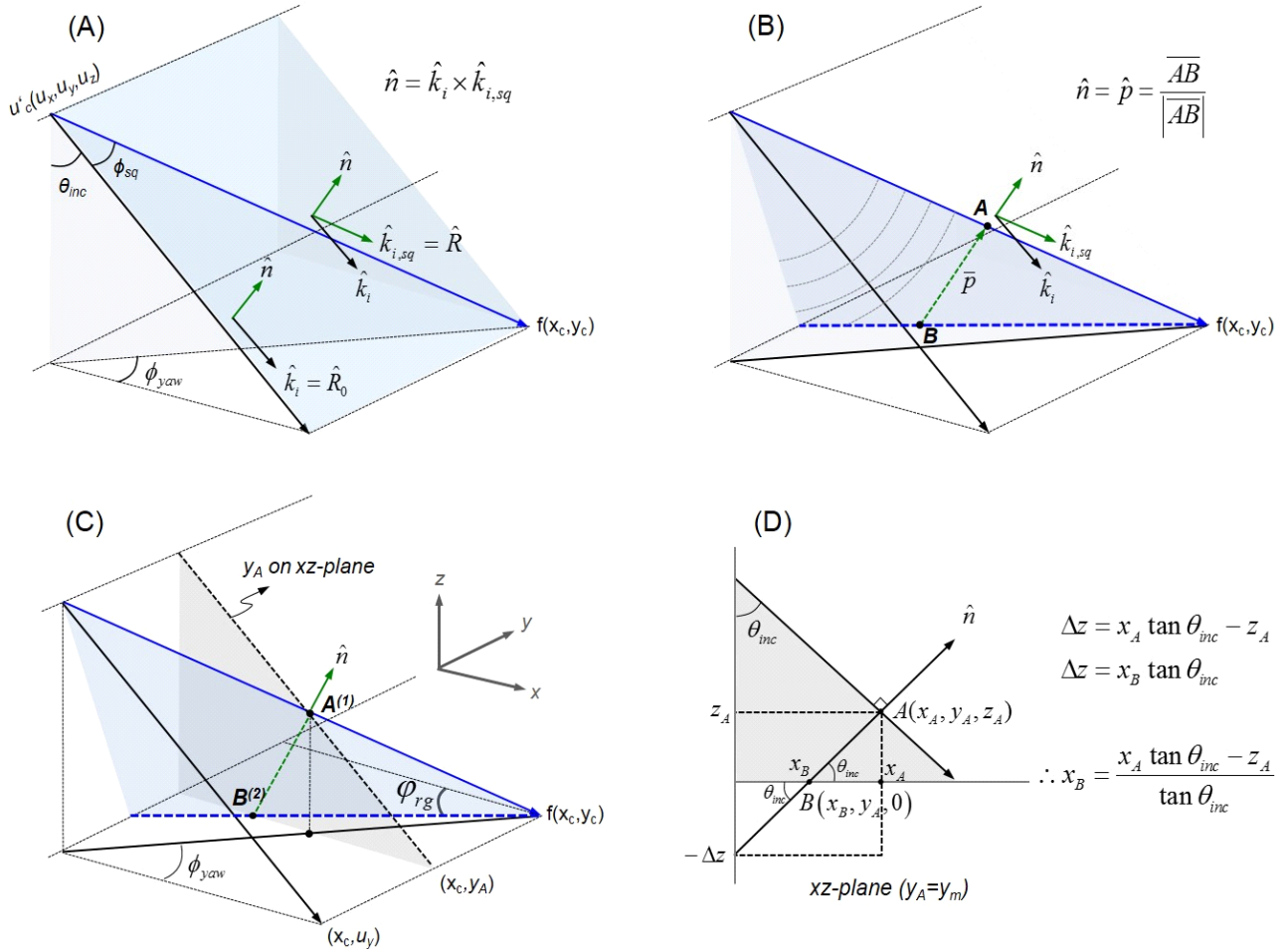
그림 4. Squint-SAR 시스템의 거리방향 성분 분석(지면에 투영된 전파 진행방향 궤적) Fig. 4. Geometry of squint-SAR system for analyzing a range component(projected trace of the propagating-wave onto ground plane).
