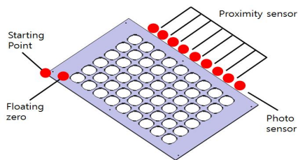
Fig. 16. Sensor position
