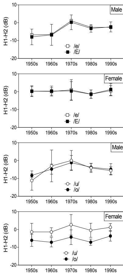
그림 7. /ㅓ/-/ㅓ/와 /ㅏ/-/ㅓ/의 평균 H1-H2 Figure 7. Mean H1-H2s of /e-/E/ and /o-/u/ with SD
