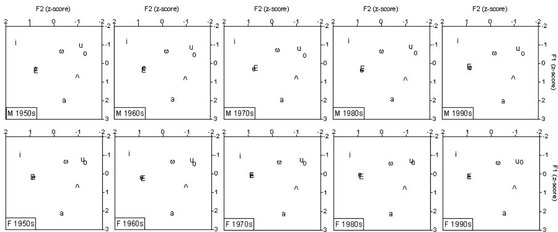
그림 2. 8모음의 F1/F2 평면 Figure 2. F1/F2 space of eight vowels
