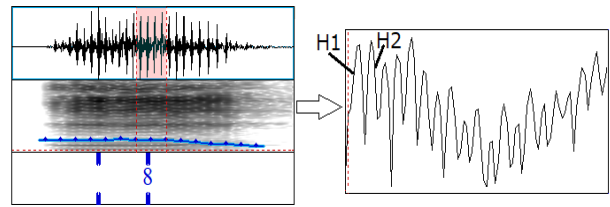
그림 1. /ㅈ/의 H1과 H2 Figure 1. H1 and H2 of /ㅈ/
