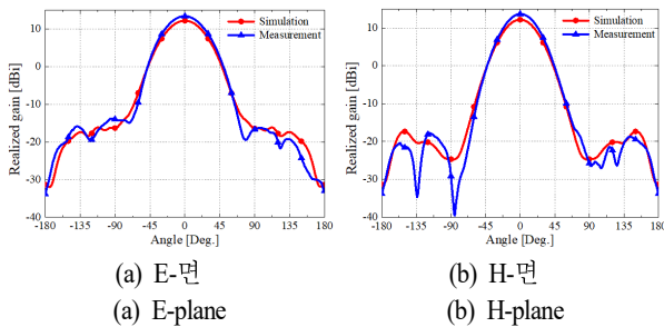
그림 7. 제안한 혼 안테나의 방사패턴 Fig. 7. Radiation pattern of the proposed horn antenna.
