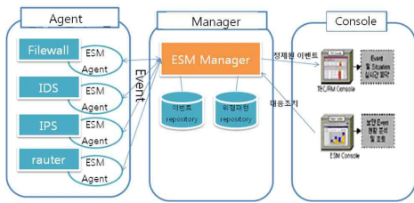
그림 3. ESM 구성 요소
