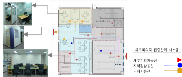
<그림 4> 형사당직조사 공간모형
