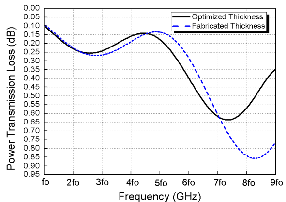
그림 2. 최적화 분석 두께와 제작 적용 두께에 대한 전파투과손실 비교 Fig. 2. Comparison of power transmission loss between optimized thickness and fabricated thickness.
