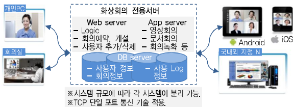
(그림 9) 포엔비VideoOffice 구성도
