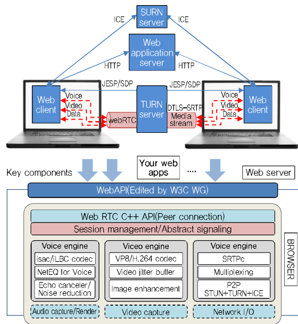
(그림 2) WebRTC아키텍처 및 연동구조
