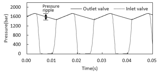
(d) Inlet and outlet valve pressure
