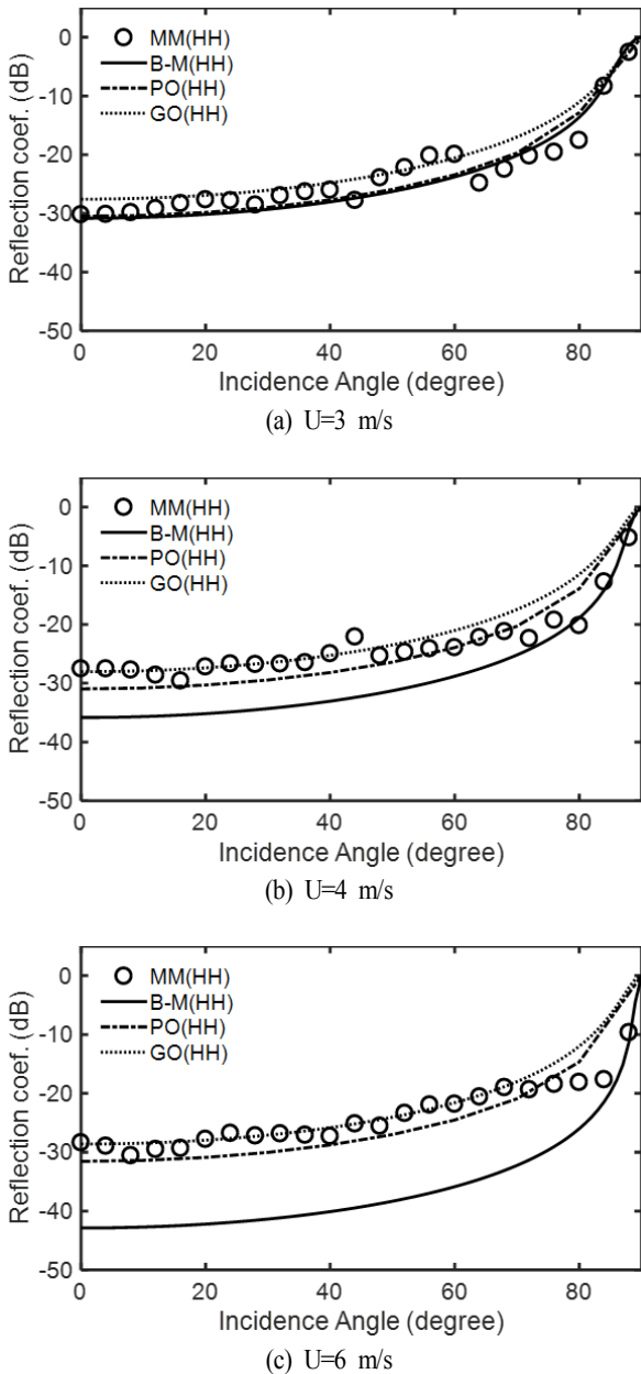
그림 4. 세 개의 풍속에 따른 비교 결과 Fig. 4. Comparisons for three different wind speeds.
