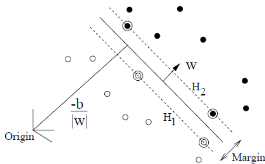
그림 3. SVM의 기본 개념 Fig. 3. The basic concept of SVM.
