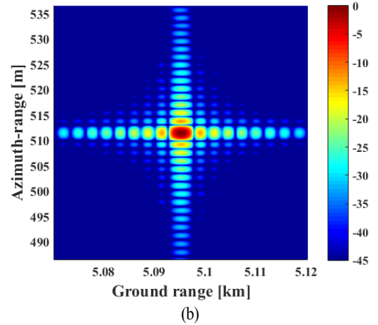
그림 7. (a) 제안된 기법으로 보상된 SAR 영상, (b) 기존의 이동 표적 보상 알고리즘으로 보상된 SAR 영상 Fig. 7. Compensated SAR images using (a) the proposed and (b) the conventional motion compensation(MOCOM) algorithms.
