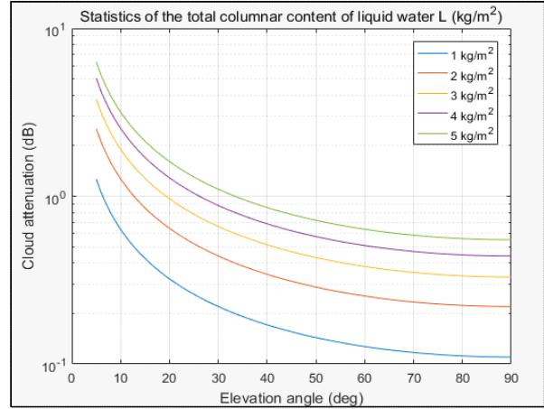
그림 4. 양각 5~90°에서의 구름감쇠(dB) Fig. 4. Cloud attenuation at elevation 5~90 deg(dB).
