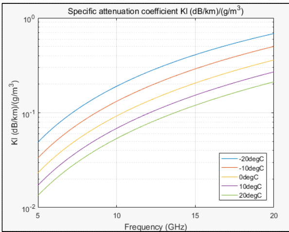
그림 3. 구름감쇠계수 Fig. 3. Specific attenuation coefficient of cloud.
