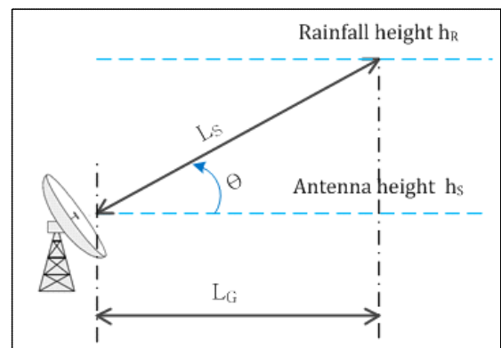
그림 1. 강우 경로의 도식적 표현 Fig. 1. Schematic representation of a rain path.
