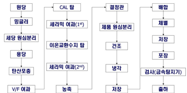
그림 1. 설탕 제조공정.
