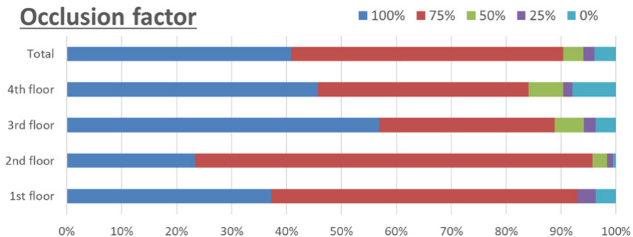
Fig. 3 The actual use of roller shades
