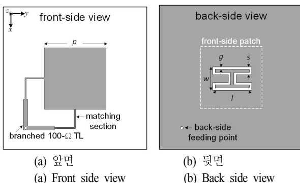
그림 1. 제안한 원형 편파 안테나 구조 Fig. 1. Configuration of the proposed circular polarized antenna.
