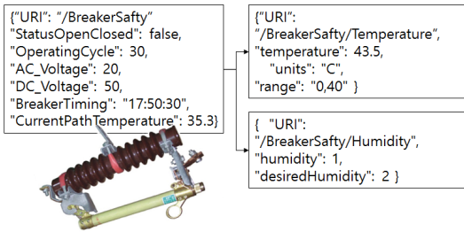
그림 5. 고압차단기에 대한 센서 정보 시험 결과 json 파일 Fig. 5. json file of high voltage breaker with temperature and humidity sensor
