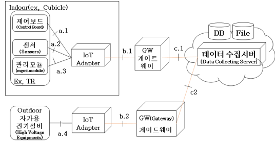
그림 2. 사물인터넷을 이용한 전기설비안전관리 인프라 구조 Fig. 2. IoT based network architecture for electrical safety management
