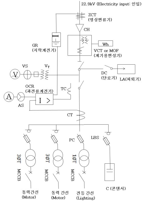
그림 1. 고압 자가용 설비 결선도 Fig. 1. IoT High-voltage equipment wiring diagram
