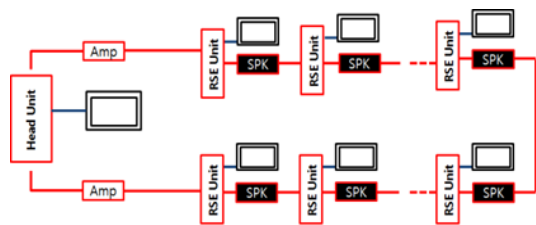
그림 3. 프리미엄 고속버스 내의 멀티미디어 시스템 전체구조 Fig. 3. Overall structure of multimedia system in premium express bus
