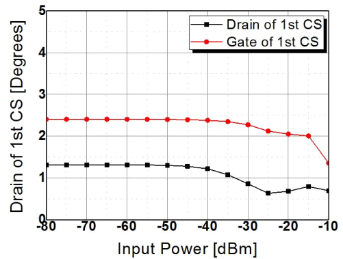
그림 8. 입력 발룬의 2차측 입력전력 대 위상차 Fig. 8. Input balun's phase difference versus input power.
