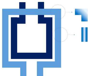
그림 2. 표피 효과에 의한 전류의 흐름 Fig. 2. The current flow by skin effect.
