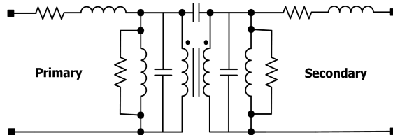
그림 3. 수동형 발룬의 모델링 Fig. 3. The modeling for passive balun.
