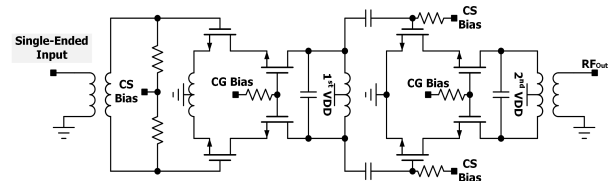
그림 5. 2단 캐스코드 차동 저 잡음 증폭기 회로도 Fig. 5. 2 stage cascode differential LNA.
