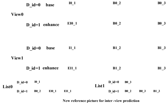
그림 2. 시점 간 예측을 지원하기 위해 설계된 참조화면리스트의 전체 구조 Fig. 2. Overall architecture of the designed reference picture list supporting inter-view prediction
