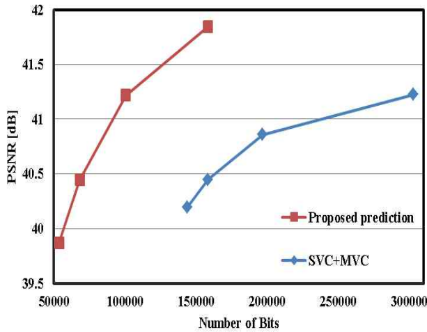
그림 4. Poznan Hall 시퀀스에 대한 PSNR 성능 비교 Fig. 4. Comparison of PSNR performance for the Poznan Hall sequence.
