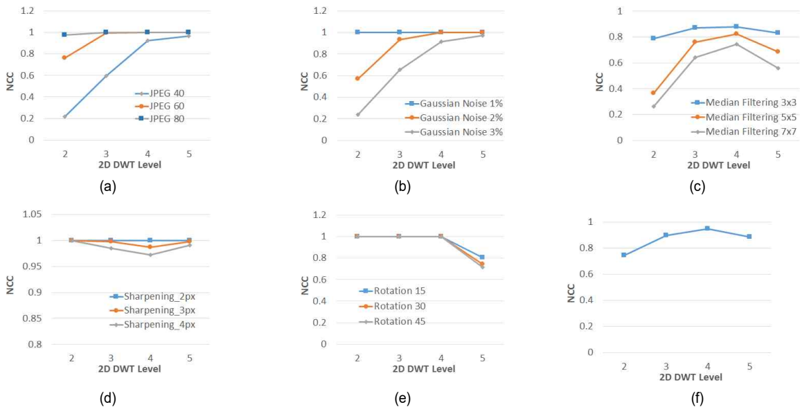
그림 9. 1,024×1,024영상의 실험 3 결과: (a) JPEG 압축 공격, (b) 미디언 필터링 공격, (c) 가우션 잡음첨가 공격, (d) 샤프닝 공격, (e) 회전 공격, (f) 모든 공격에 대한 평균
