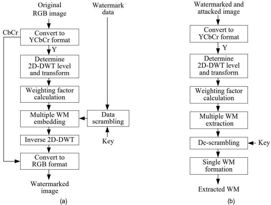
그림 11. 제안하는 DWM 방법: (a) WM 삽입과정, (b) WM 추출과정. Fig. 11. The proposed DWM scheme: (a) WM embedding procedure, (b) WM extracting procedure.
