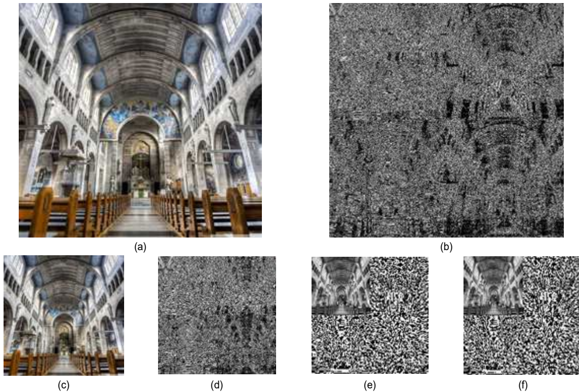
그림 2. 2D-DWT의 예: (a) 1,024×1,024 원영상, (b) (a)를 4-레벨 2D-DWT 결과, (c) (a)를 512×512로 다운-샘플링한 영상, (d) (b)를 3-레벨 2D-DWT 한 결과, (e) (b)의 레벨-4 네 부대역, (f) (d)의 레벨-3 네 부대역 Fig. 2. An example of 2d-DWT: (a) 1,024×1,024 original image, (b) result from 4-level 2D-DWT for (a), (c) 512×512 down-sampled result from (a), (d) result from 3-level 2D-DWT for (c), (e) four level-4 subbands of (b), (f) four level-3 subbands of (d).
