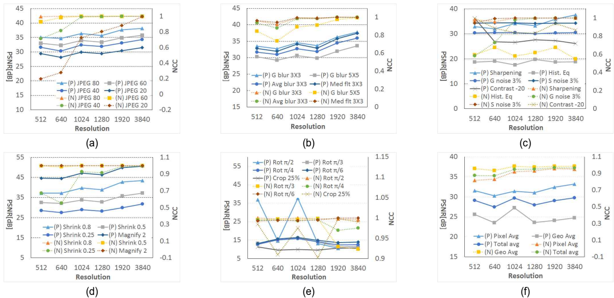
그림 13. 공격에 대한 실험결과: (a) JPEG 압축, (b) 가우시안 블러링, 평균 블러링, 미디언 필터링, (c) 샤프닝, 히스토그램 평활화, 가우시안 잡음첨가, Salt&pepper 잡음첨가, 콘트라스트 조정, (d) 스케일링(축소, 확대), (e) 회전, cropping, (f) 평균들.
