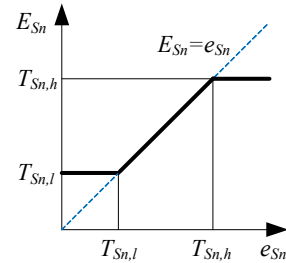
그림 8. 양자화 범위 Fig. 8. Quantization range
