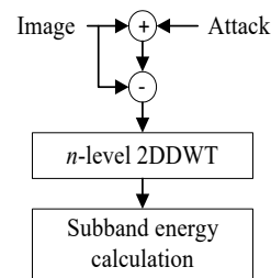
그림 7. 공격의 영향을 측정하기 위한 실험 Fig. 7. Experiment to estimate the effect of an attack
