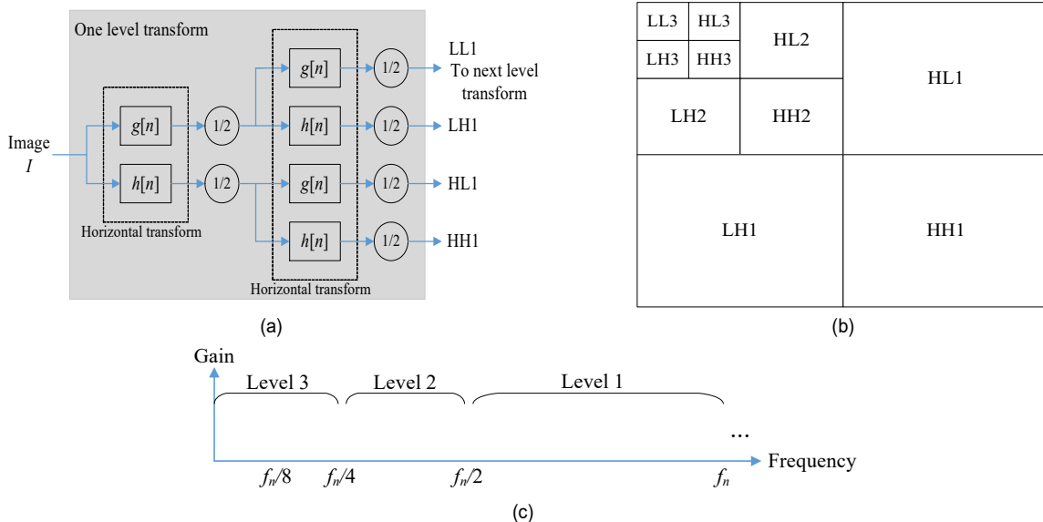
그림 1. 2D-DWT와 부대역의 주파수 대역: (a) 필터뱅크, (b) 3-레벨 2D-DWT의 부대역, (c) 3-레벨 DWT의 주파수 대역. Fig. 1. 2D-DWT and the frequency band of subbands: (a) filter bank, (b) subbands after 3-level 2D-DWT, (c) frequency band for 3-level DWT.
