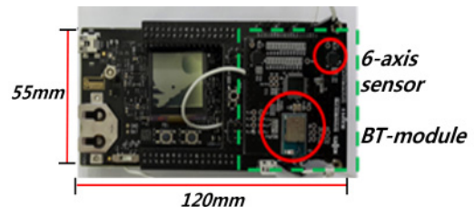
그림 5. 웨어러블 디바이스 플랫폼 Fig. 5. Wearable device platform
