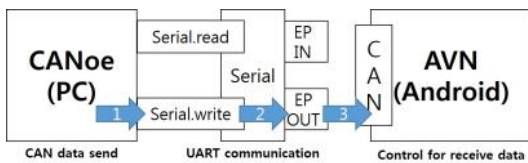
그림 3. CAN 데이터 수신구조 Fig. 3. CAN data reception structure
