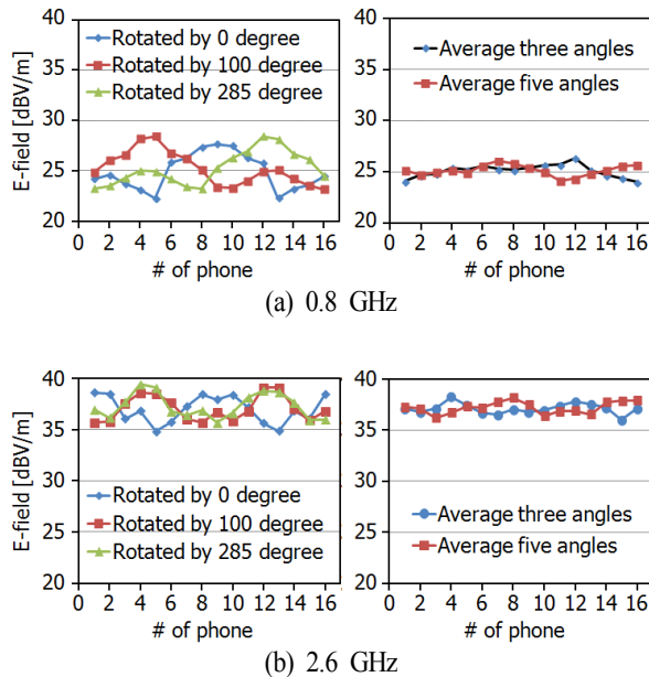
그림 8. 회전각도에 대한 평균값을 이용하여 단말기 간 전기장 균일도 개선 Fig. 8. Uniformity improvement by using average value among rotation angles.
