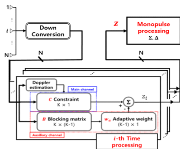
그림 1. GSC 기반의 모노펄스 시스템 블록도 Fig. 1. GSC based monopulse system block diagram.
