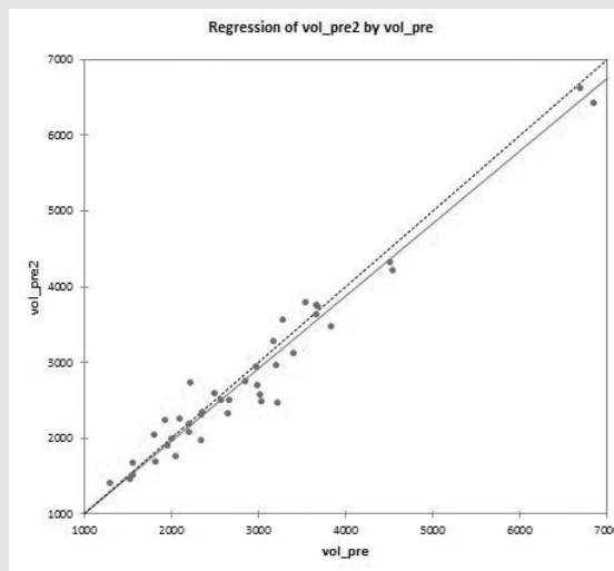
그림 16. 엑셀에서 Passing and Bablok regression 을 실행한 결과
