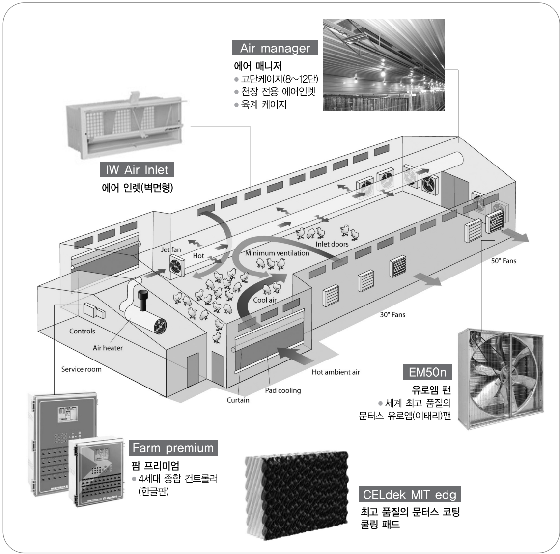
▲ 문터스의 양계 환기 시스템
